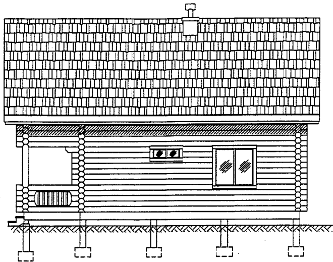
RIGHT ELEVATION
